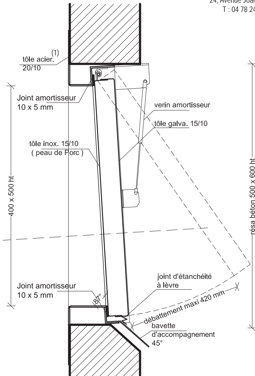
VUE EN COUPE échelle 1/5°
